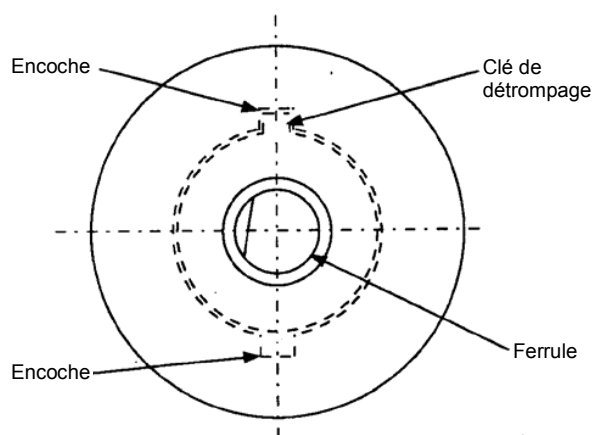
Figure 3 – Exemple de support de connecteur
