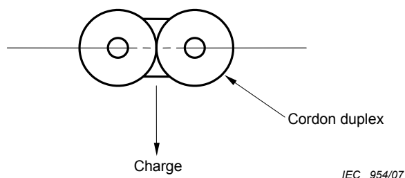
Figure 2 – Application de la charge dans le cas d'un cordon duplex
