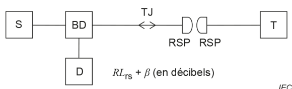
Figure 2 – Montage de mesure pour RSC accouplés
