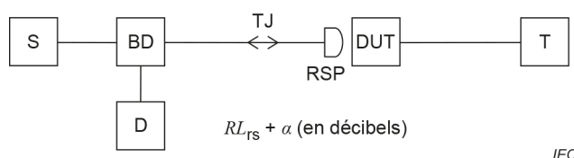
Figure 4 – Montage de mesure pour essai de sélection des fibres amorce
