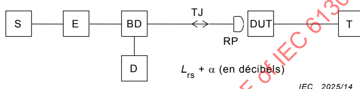
Figure 4 – Montage de mesure pour essai de sélection des connecteurs à fibres amorces
