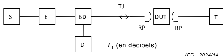
Figure 3 – Montage de mesure pour essai de sélection des connecteurs montés sur cordons
