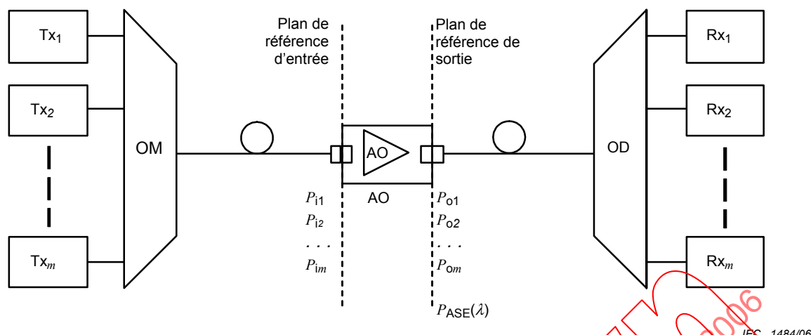
Figure 2 – Amplificateur optique dans une application à canaux multiples
