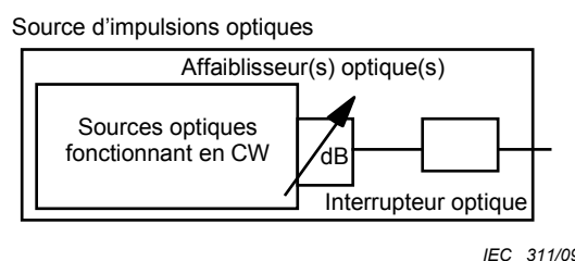
Figure 2a – Disposition avec interrupteur optique externe
