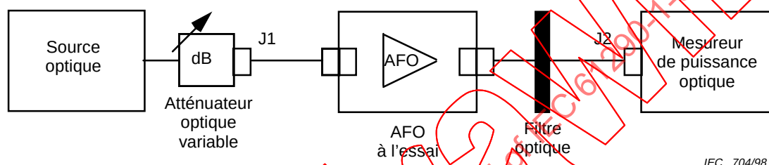
Figure 1b - Mesure de la puissance du signal de sortie et de l'ESA
