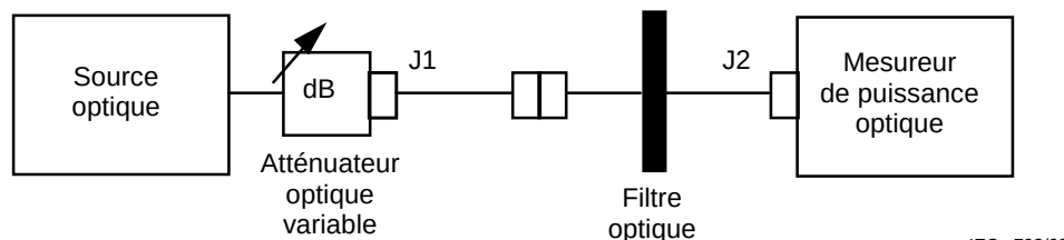
Figure 1a - Mesure de la puissance du signal d'entrée
