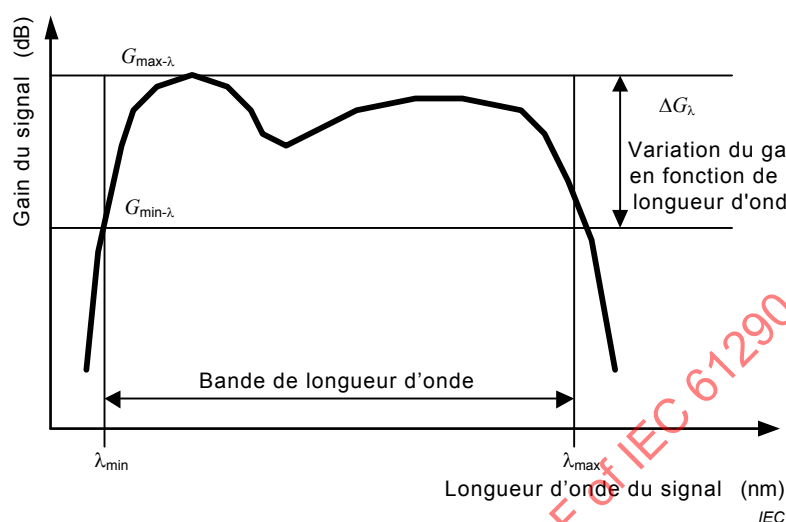
Figure 4 – Comportement typique du gain en fonction de la longueur d'onde
