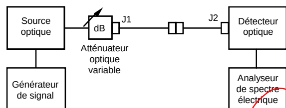
Figure 1b - Mesure de la puissance électrique modulée du signal d'entrée
