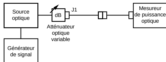
Figure 1a - Mesure de la puissance optique du signal d'entrée moyennée dans le temps
