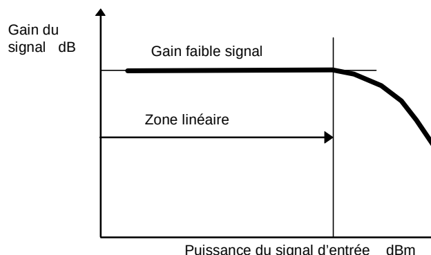
Figure 2 – Variation typique du gain en fonction de la puissance du signal d'entrée
