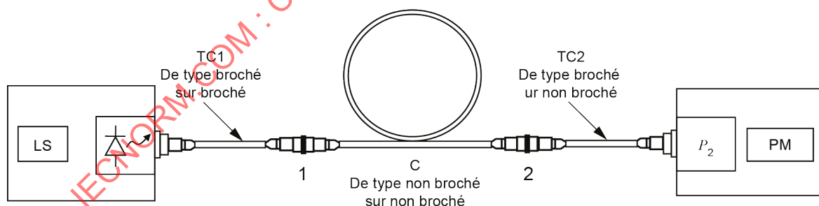
Figure A.7 – Mesurage de référence pour le câblage de type non broché sur non broché au moyen d'un mesureur de puissance broché
