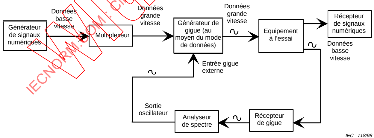
Figure 3 – Configuration pour la mesure de la fonction transfert de gigue – technique par démultiplexage
