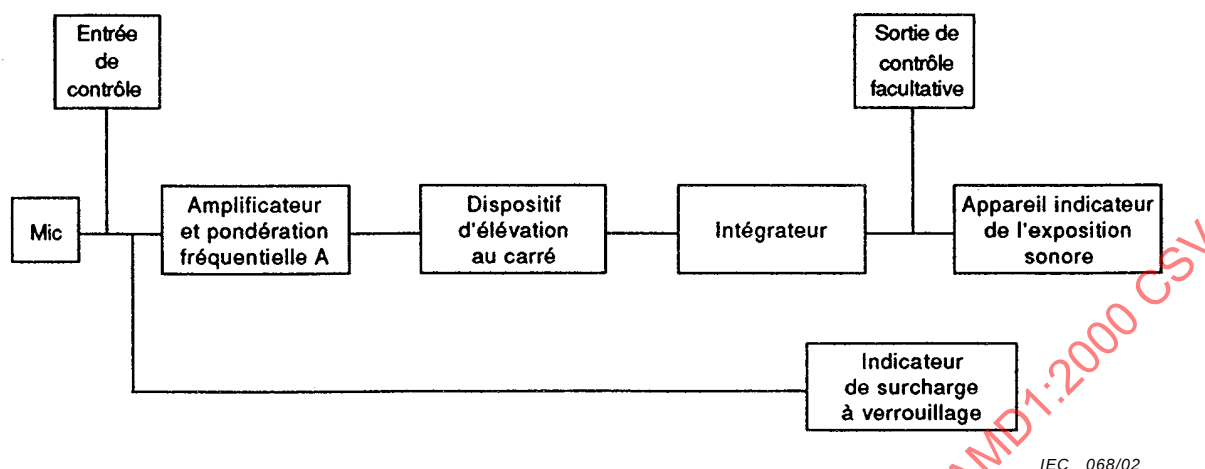
Figure 1 – Eléments fonctionnels d'un exposimètre acoustique individuel
