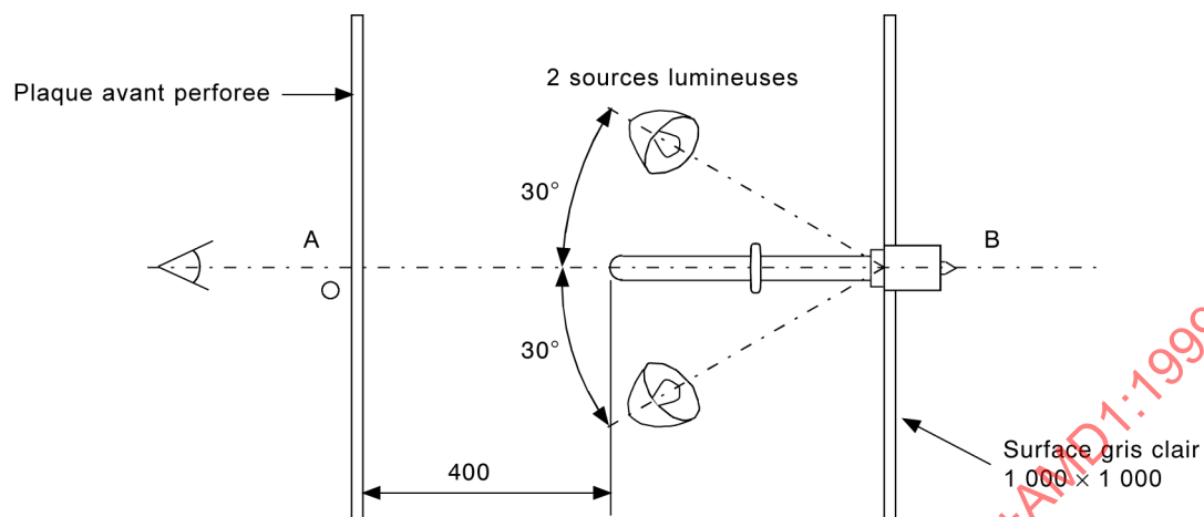
Figure 4a – Vue du dessus
