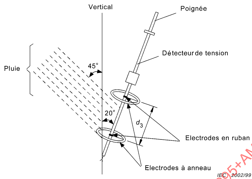
Figure 8 – Disposition pour mesurage de protection de contournement pour détecteur de type extérieur
