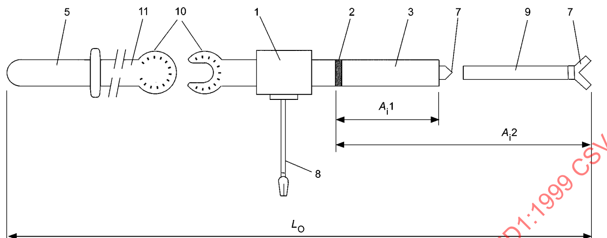
Figure 1c – Détecteur en élément séparé avec une perche isolante adaptable
