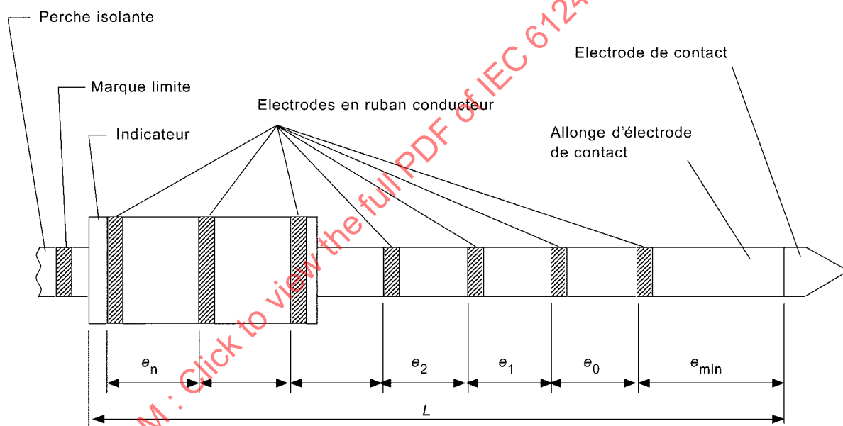
Figure 11 – Montage d'essai pour rigidité diélectrique pour boîtier indicateur et élément résistif
