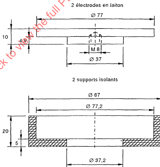
Figure C.3 – Plan d'exécution des accessoires pour électrode et support d'électrode
