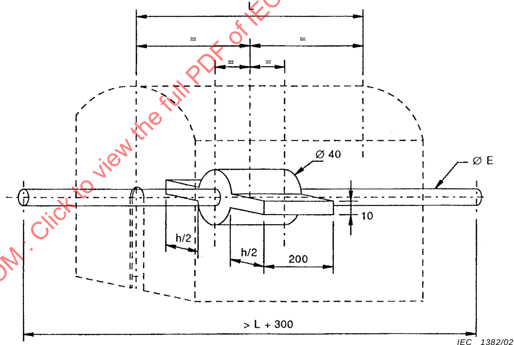
Figure E.3 – Electrode pour protecteur d'isolateur rigide
