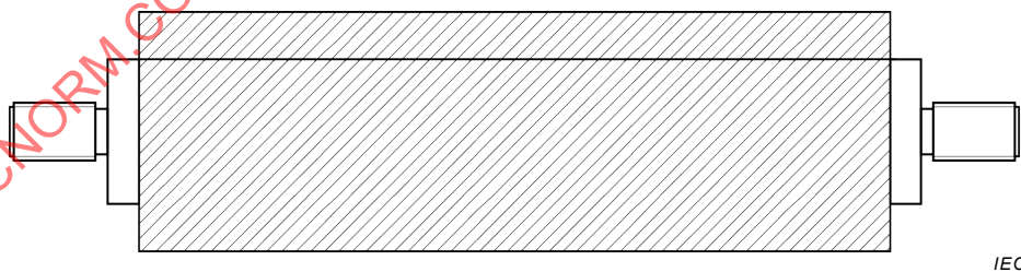
Figure 11 – Appareil d'essai – Vue latérale
