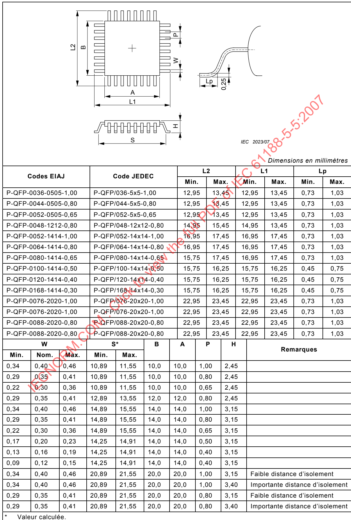
Figure 2 – Dimensions des composants à boîtier PQFP (carré)
