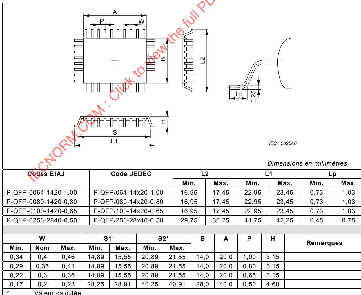
Figure 6 – Dimensions des composants à boîtier PQFP (rectangulaire)
