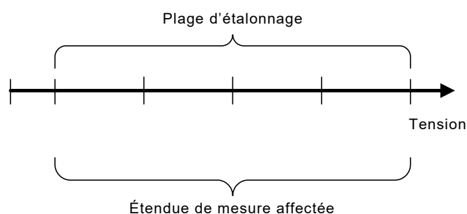
Figure 2 – Étalonage par comparaison sur la plage de pleine tension
