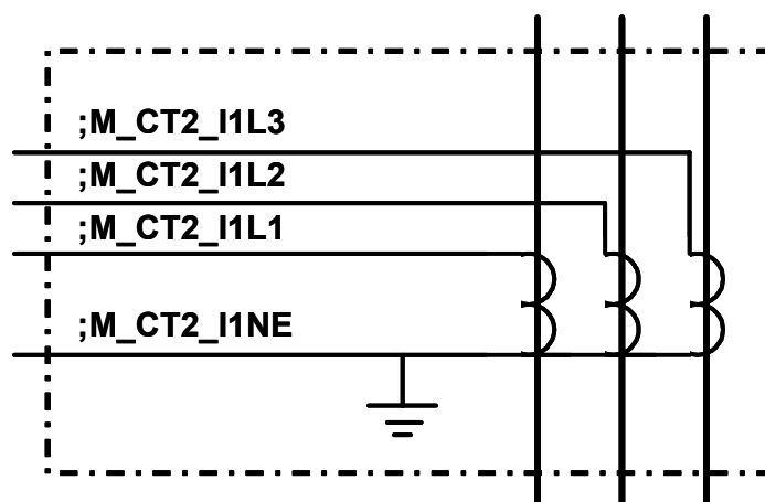
Figure 5 – Exemple de signaux de mesure
