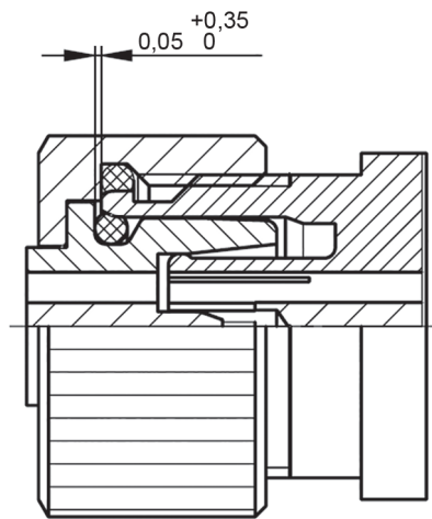
Figure 4 – Connecteur de type manuel à vis
