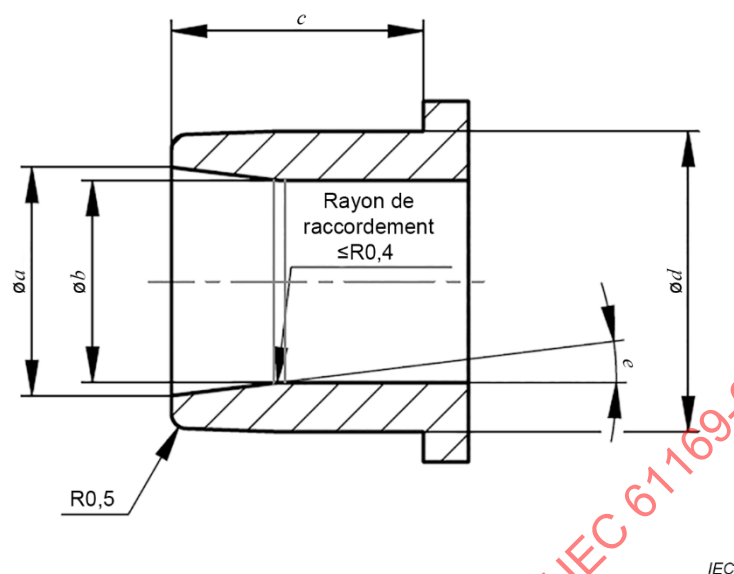
Figure 7 – Bagues calibrées pour contact extérieur femelle (pour les dimensions, voir le Tableau 4)
