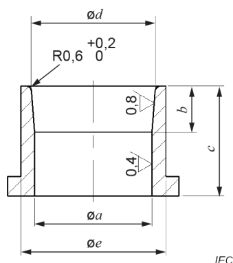
Figure 4 – Bague de calibre pour le contact extérieur de fiche
