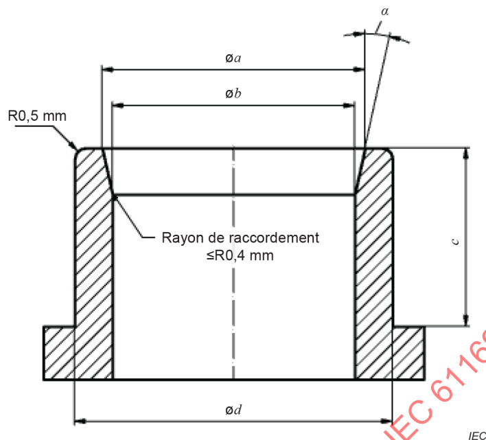
Figure 7 – Bagues calibrées pour contact extérieur femelle (pour les dimensions, voir Tableau 4)
