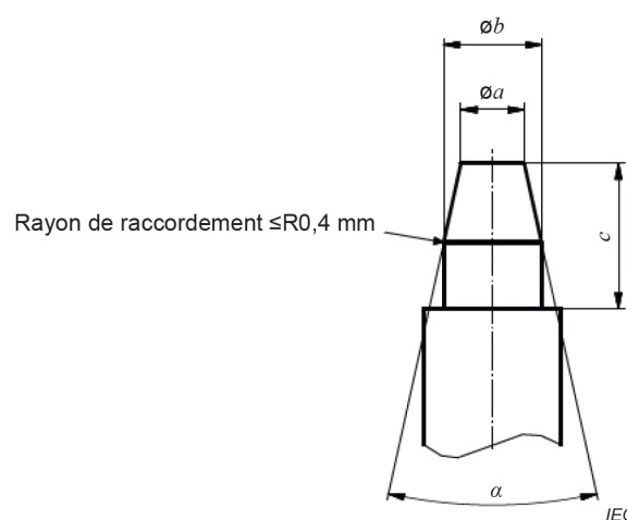
Figure 6 – Broches calibrées pour contact central femelle (pour les dimensions, voir Tableau 3)
