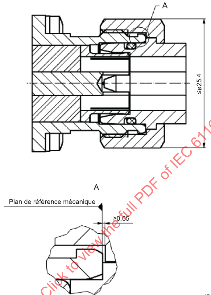
Figure 3 – Couplage de type à vis
