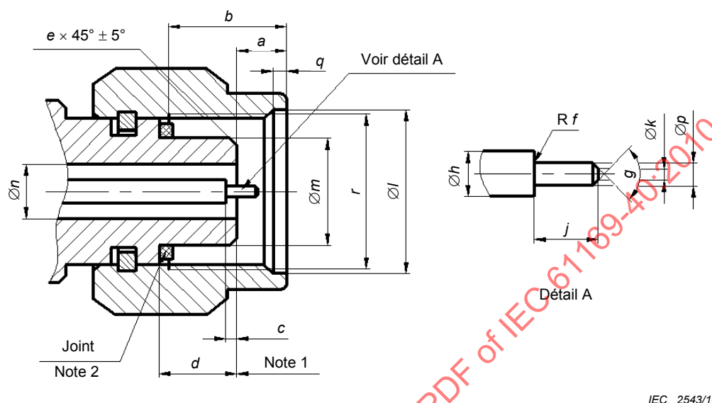
Figure 1 – Connecteur avec contact central mâle (pour les dimensions et les notes, voir le Tableau 1)
