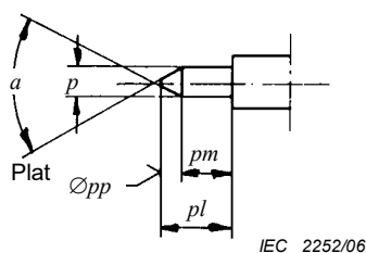
Figure 6 – Broches mâles de calibrage et d'essai pour les contacts centraux femelles (pour les notes et les dimensions, voir le Tableau 3)
