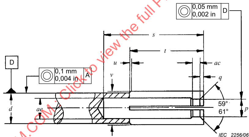
Figure 10 – Détails du contact central femelle (pour les notes et les dimensions, voir le Tableau 5)
