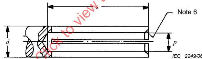
Figure 4 – Détails du contact central femelle (pour les notes et les dimensions, voir le Tableau 2)
