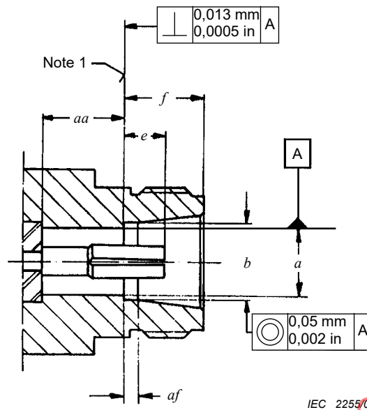
Figure 9 – Connecteur de référence avec contact central femelle (pour les notes et les dimensions, voir le Tableau 5)
