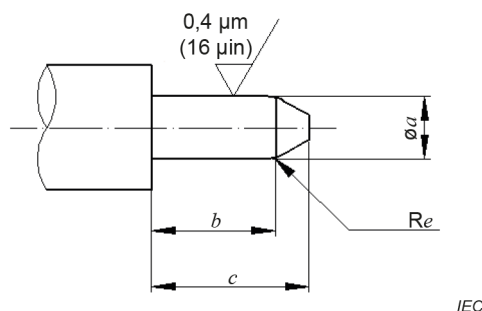
Figure 3 – Broche calibrée pour contact central femelle
