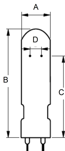
a) Tube à décharge en quartz, arc transversal
