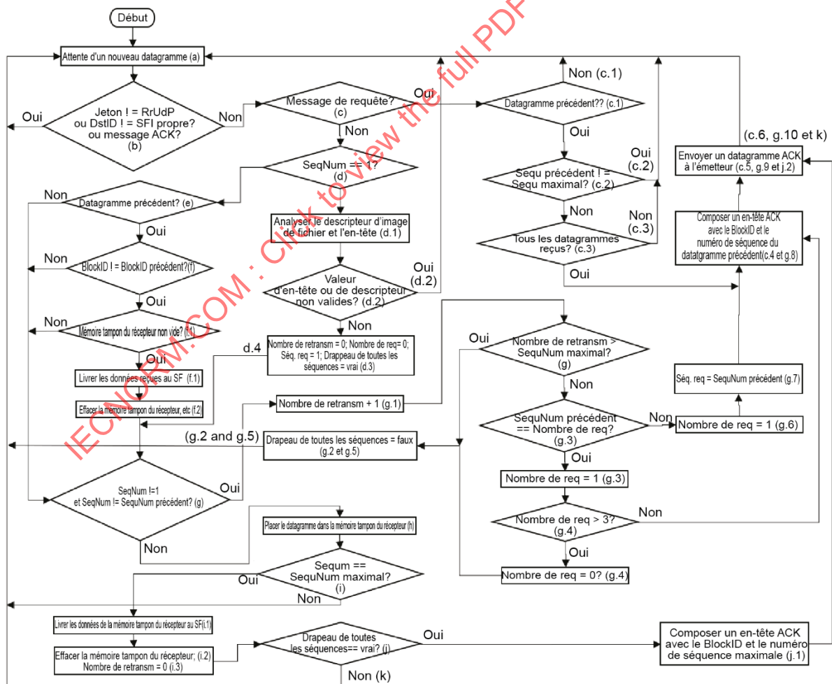
Figure 7 – Processus de réception retransmissible
