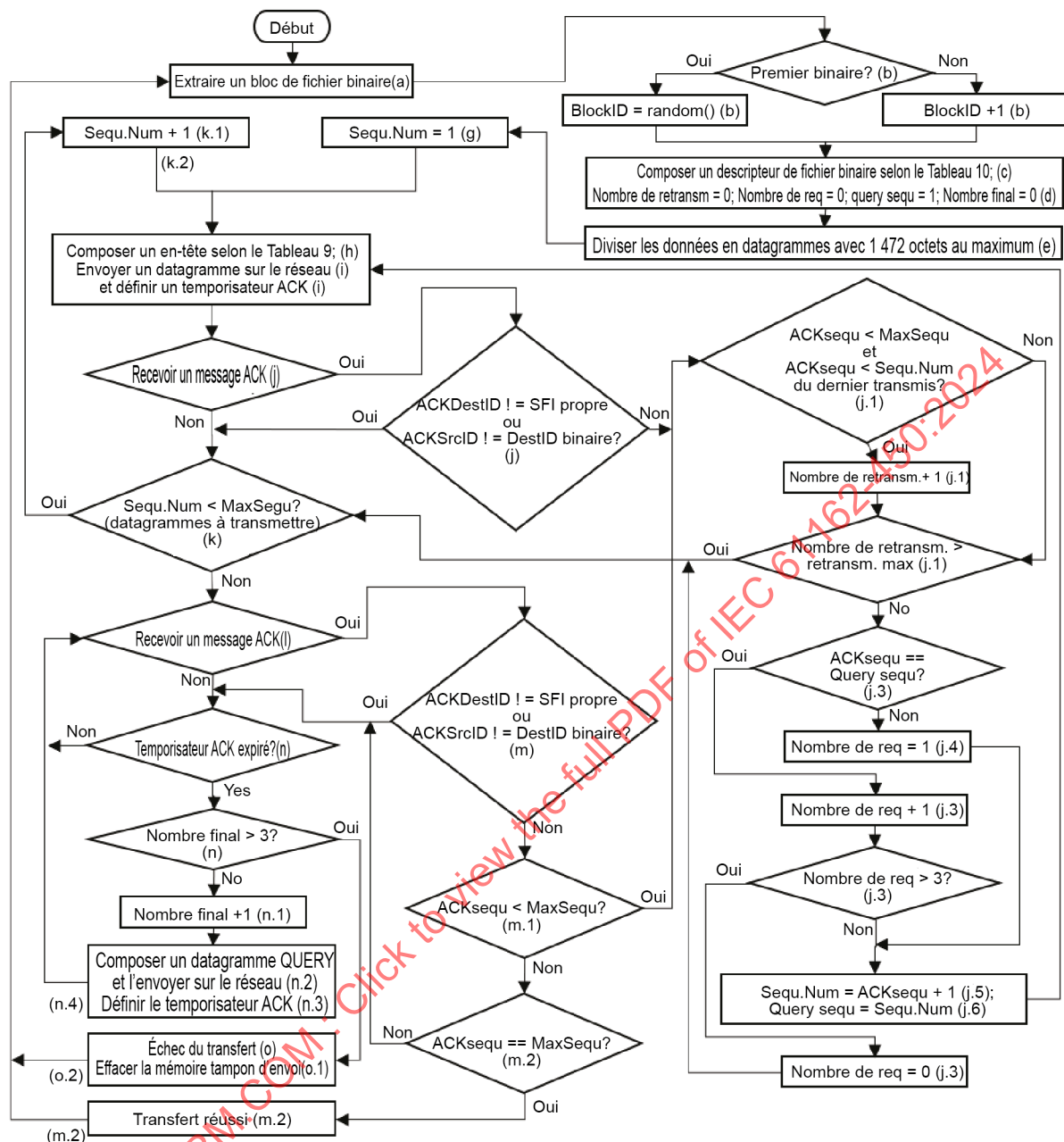
Figure 6 – Processus d'envoi retransmissible
