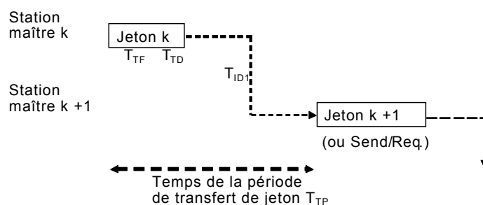
Figure 11 – Période de transfert de jeton
