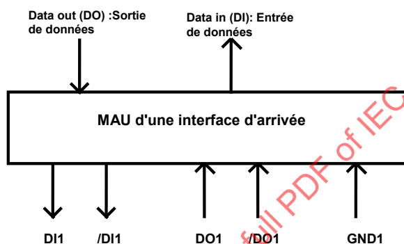
Figure 118 – MAU d'une interface d'arrivée
