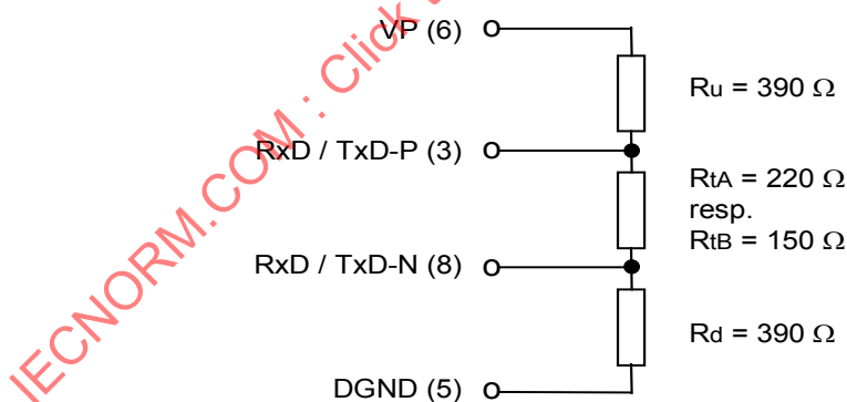
Figure 101 – Terminateur de bus
