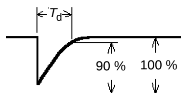
Figure 7 – Réponse caractéristique (2)
