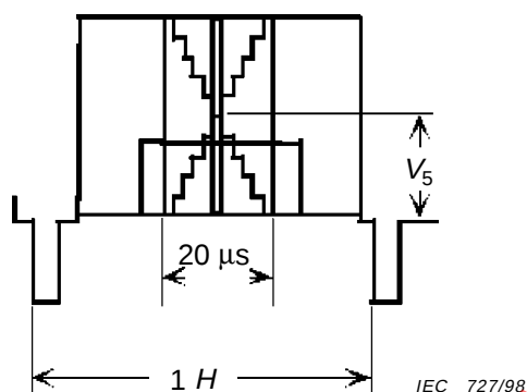
Figure 4 – Forme d'onde d'une ligne pour \bar{B} = 77 \%
