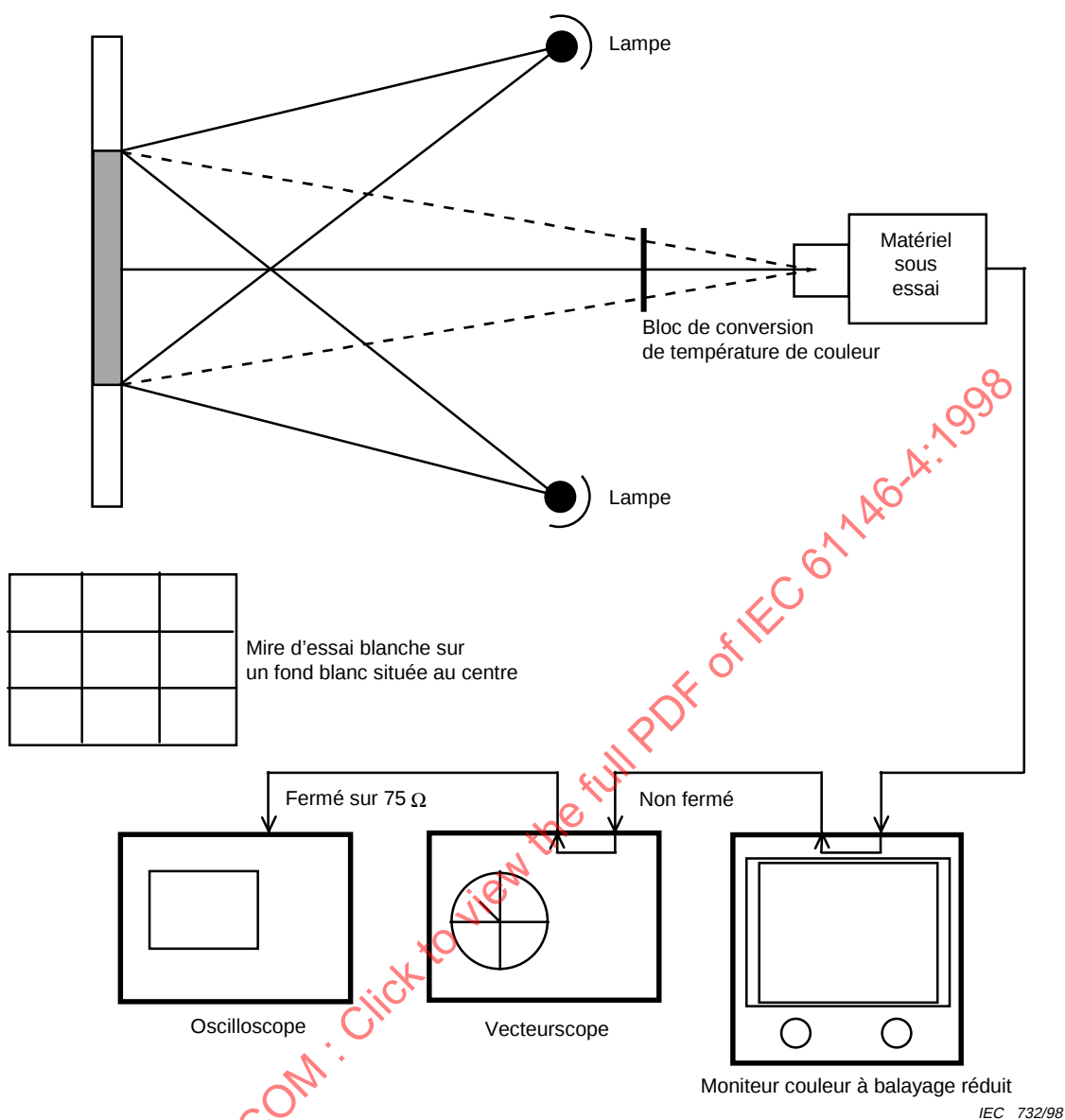
Figure 9 – Circuit de mesure de la balance automatique des blancs
