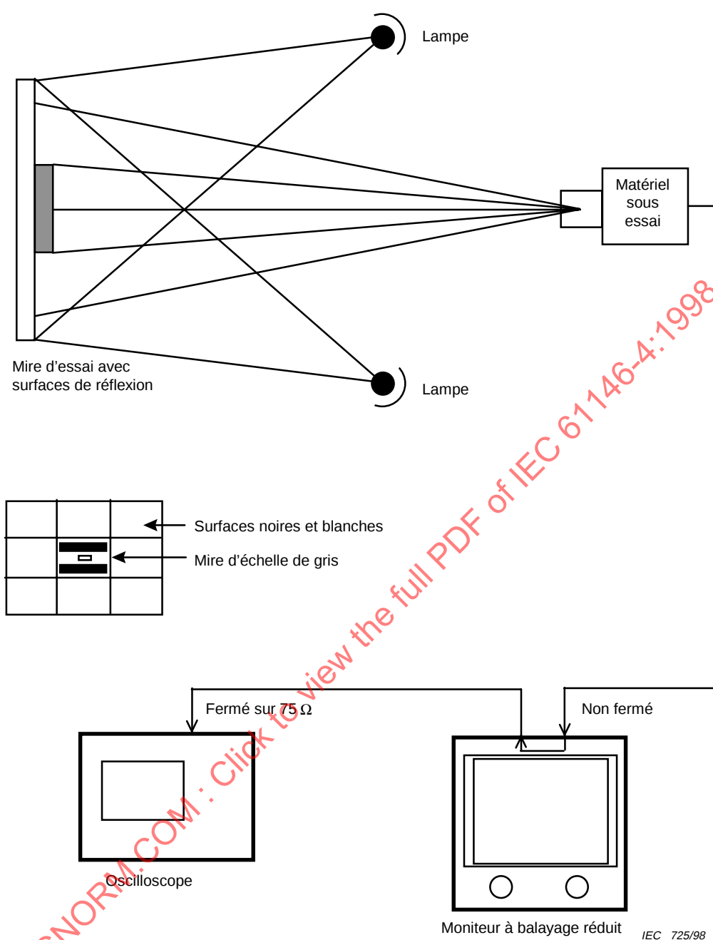
Figure 2 – Circuit de mesure pour déterminer l'influence de la luminosité moyenne
