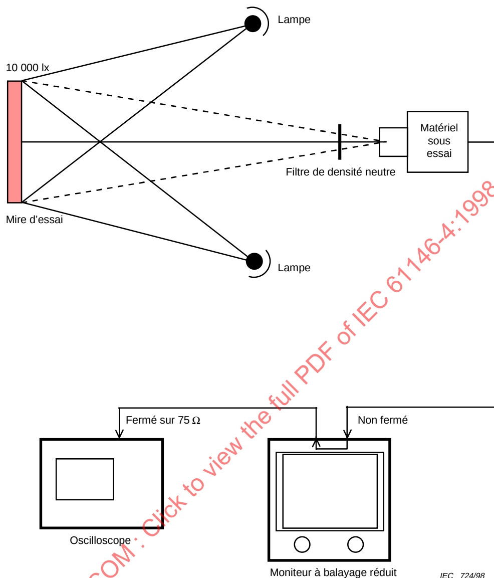
Figure 1 – Circuit de mesure pour déterminer l'influence du niveau d'éclairement
