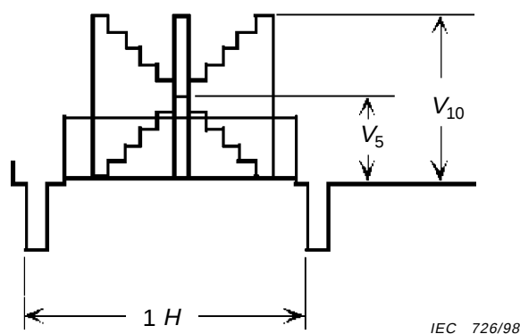
Figure 3 – Forme d'onde d'une ligne pour \bar{B} = 27 \%
