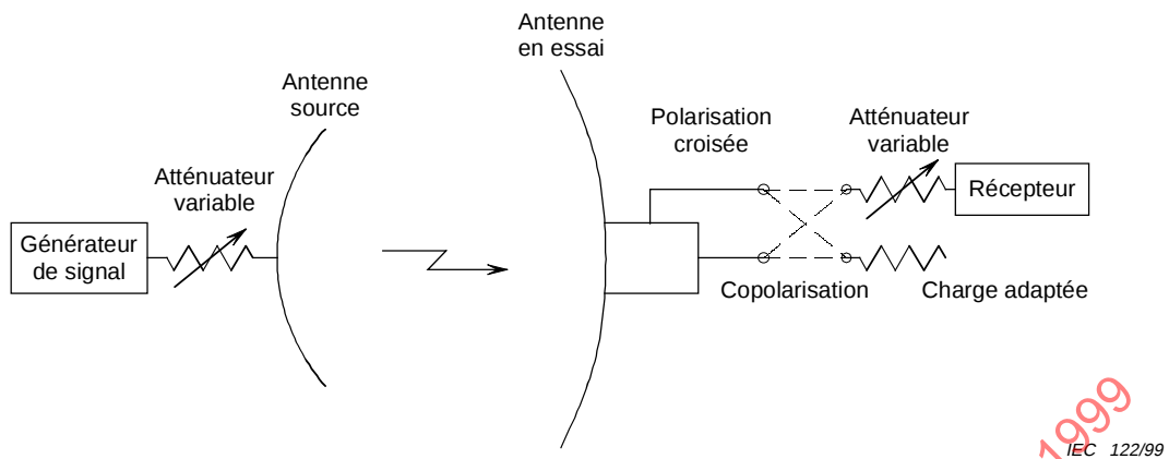
Figure 12a – Antenne à faisceau simple
