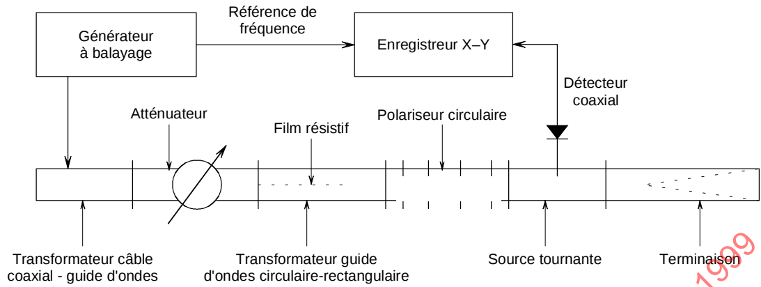
Figure A.4 – Méthode de mesure du rapport d'axes
