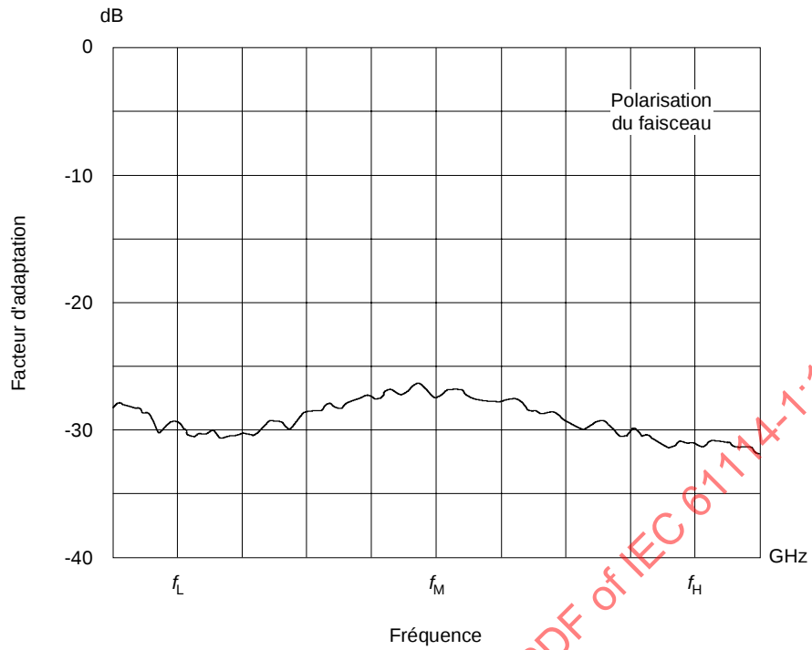
Figure 7 – Représentation graphique de l'adaptation d'impédance
