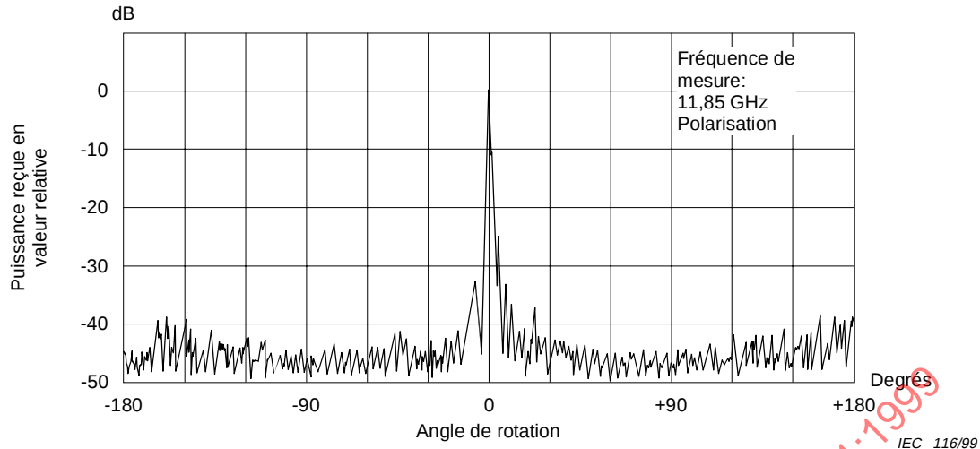
Figure 9a – Diagramme de rayonnement pour un angle important
