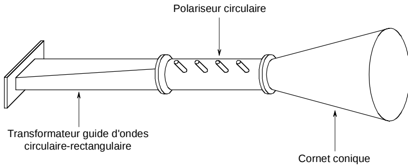
Figure A.1 – Antenne de référence à polarisation circulaire
