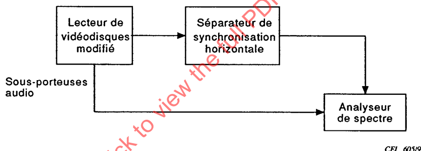
Figure N.1 – Schéma synoptique du dispositif de mesure
