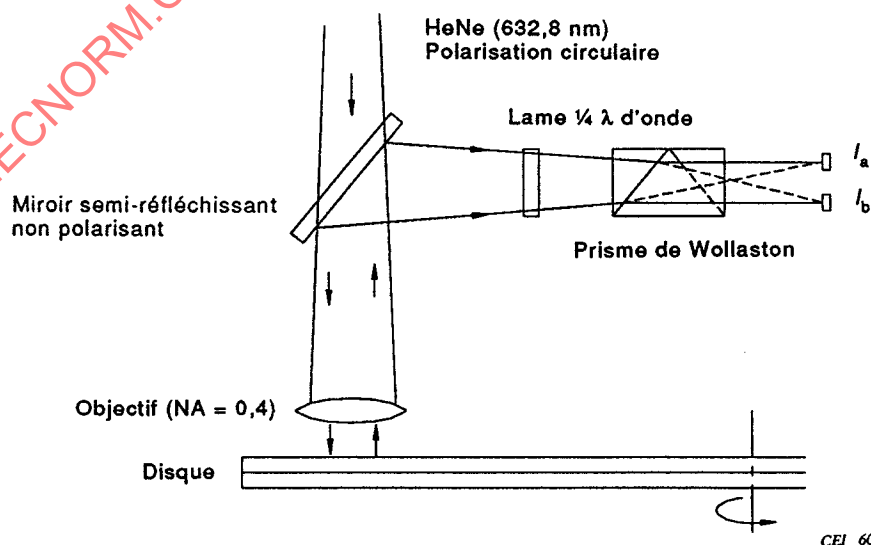
Figure L.1 – Dispositif de mesure
