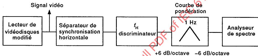
Figure K.1 – Schéma synoptique du dispositif de mesure
