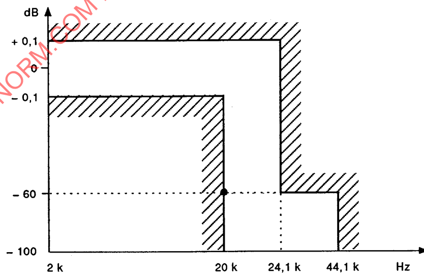
Figure 1 - Tolérances du filtre passe-bas
