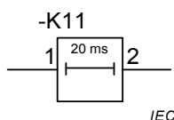
Figure 28 – Exemple de données techniques représentées à l'intérieur d'un symbole
