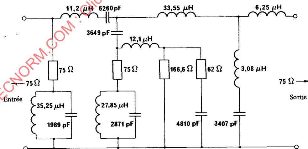
Figure 13 – Exemple de filtre de différenciation
