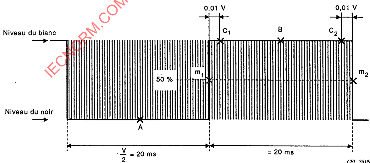
Figure 11 – Mesure des distorsions basse fréquence
