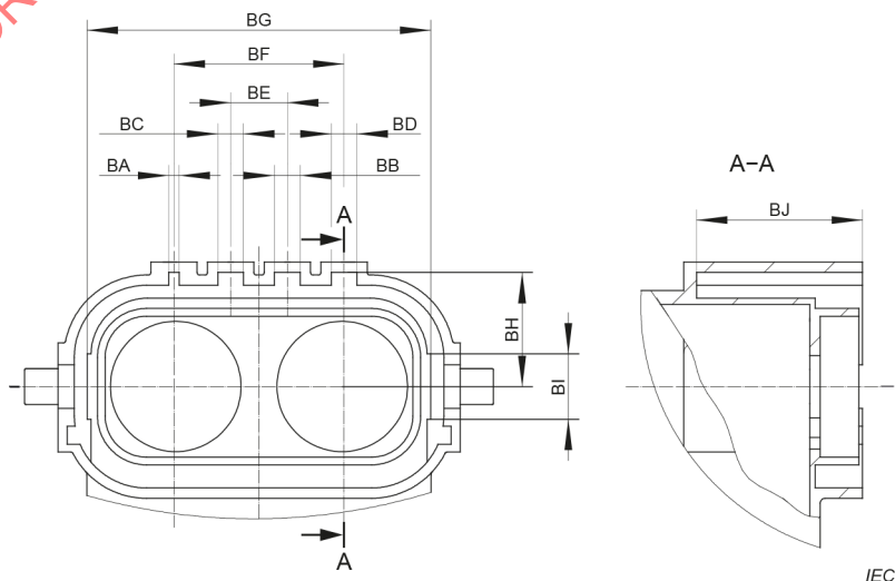
Figure 4 – Détrompages des fiches
