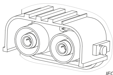
Figure 2 – Vue isométrique d'une embase
