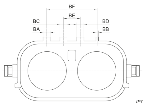
Figure 6 – Détrompages des embases
