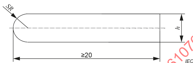
Figure 8 – Calibre pour contacts d'alimentation
