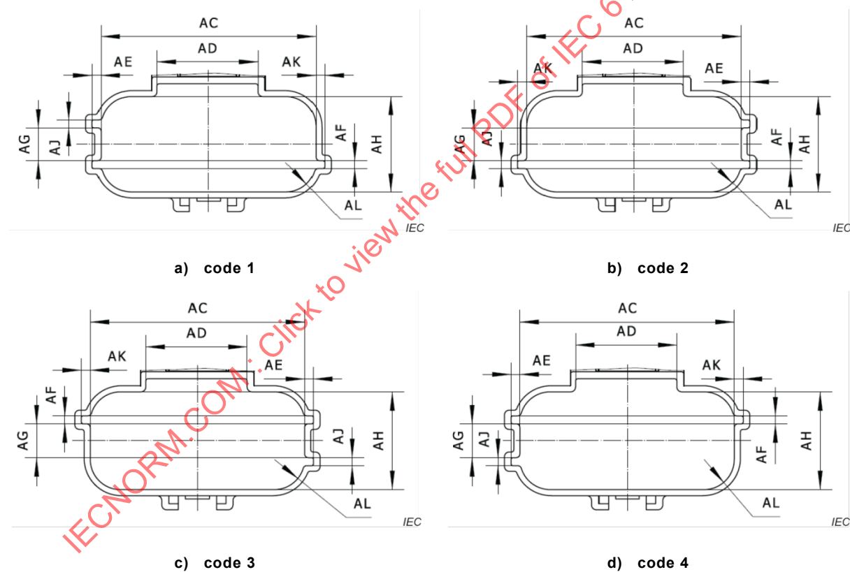
Figure 8 – Détrompage des fiches
