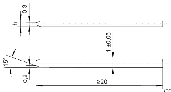
Figure 9 – Calibre pour contact de signalisation
