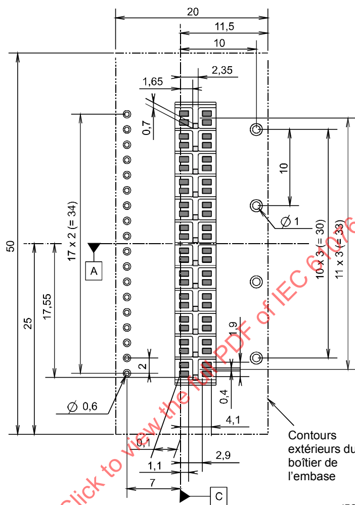
Figure 19 – Implantation sur fond de panier pour l'embase montée en CIF et en compression
