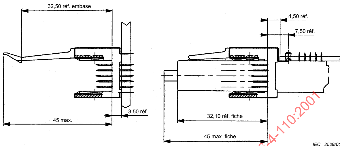
Figure 9 – Dimensions en profondeur
