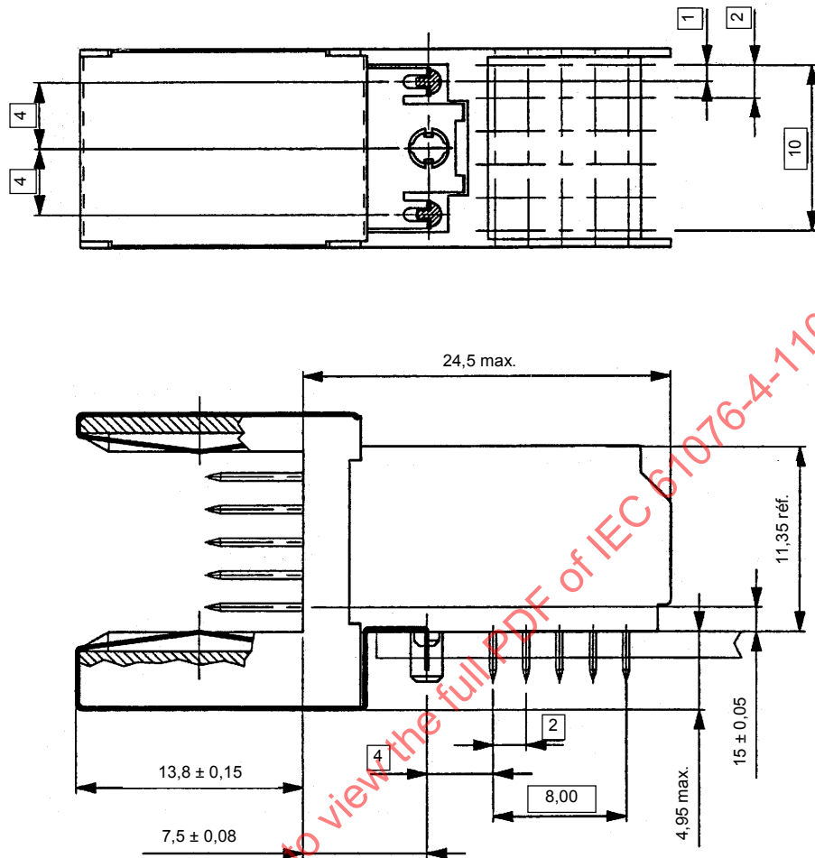
Figure 14 – Dimensions particulières aux embases à picots soudés
