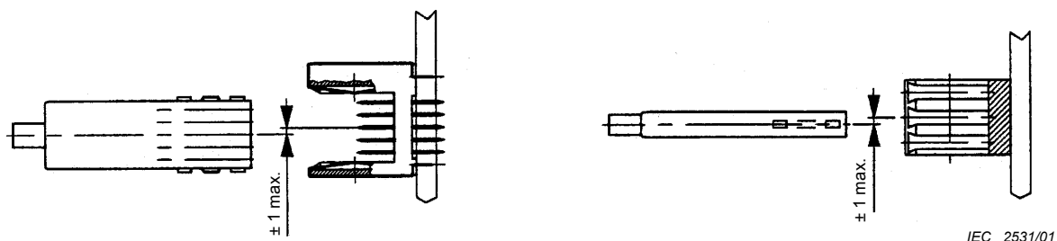
Figure 11 – Défaut d'alignement permis en largeur et en hauteur
