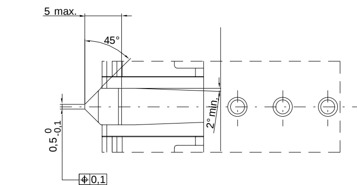
Section OP
