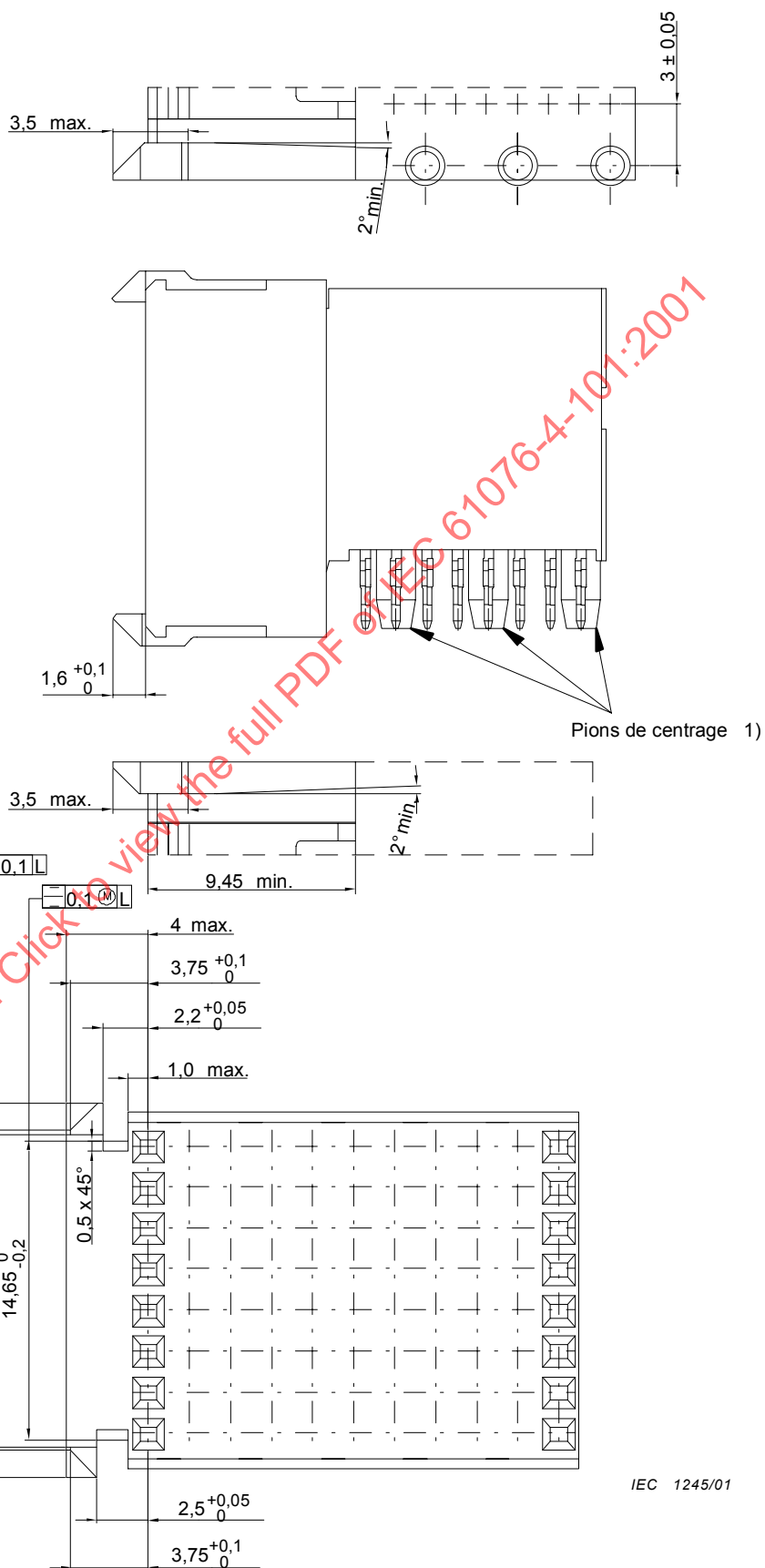
Figure 36 – Dimensions du modèle F, module de fiche d'extension 25 mm (huit rangées)
