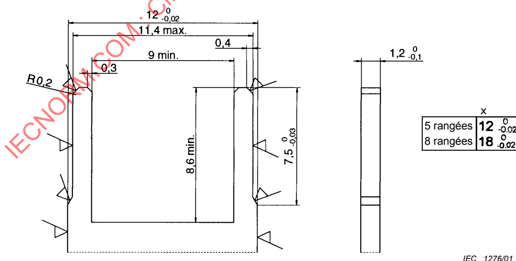
Figure 65 – Calibres de forçage et de force de rétention pour contacts femelles
