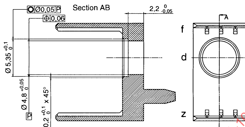
Figure 23 – Dimensions des alvéoles d'embase pour contacts spéciaux
