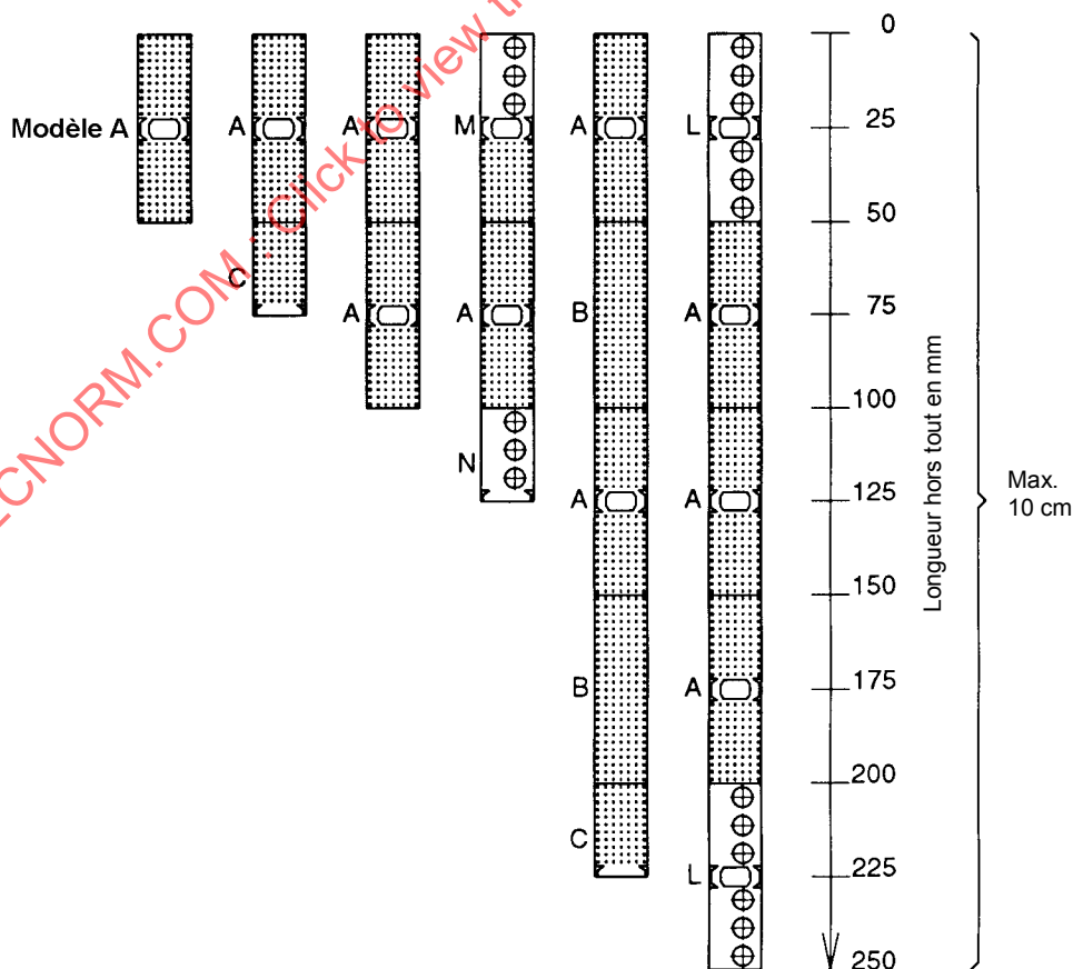
Figure 2 – Exemples de compositions de connecteurs complets
