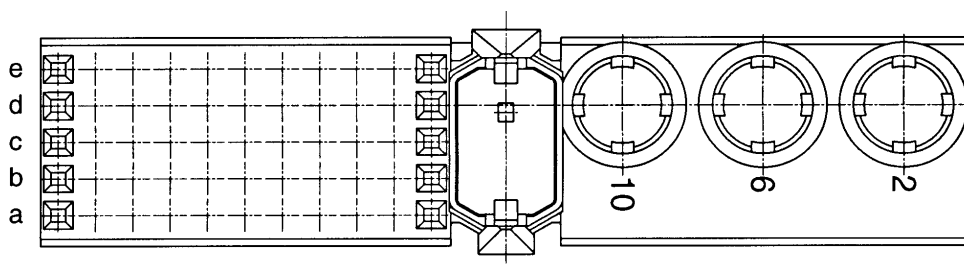
Figure 39 – Dimensions du modèle M, module de fiche mixte 50 mm avec trois contacts spéciaux
