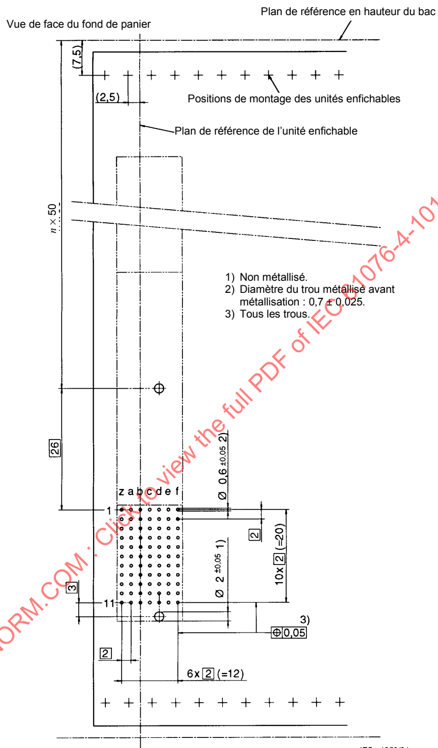
Figure 49 – Plan de perçage du fond de panier pour le modèle C
