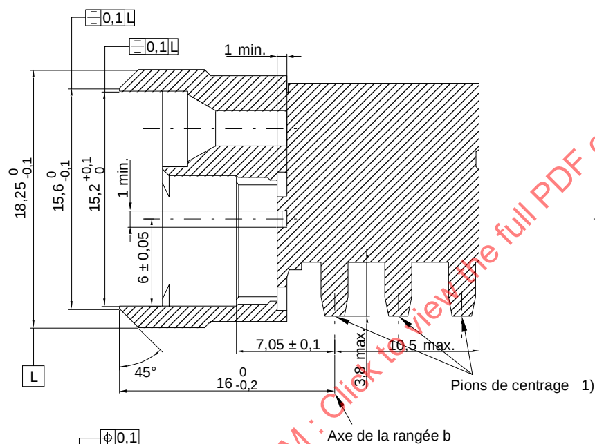
Section OP
