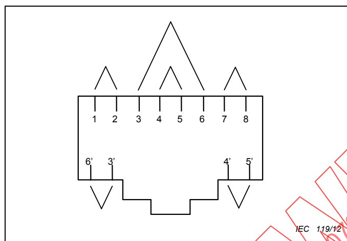
Figure 3 – Affection de groupement de broches et de paires pour embases (vue de face du connecteur)
