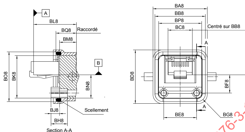
Figure 14 – Fiche, Variante 07
