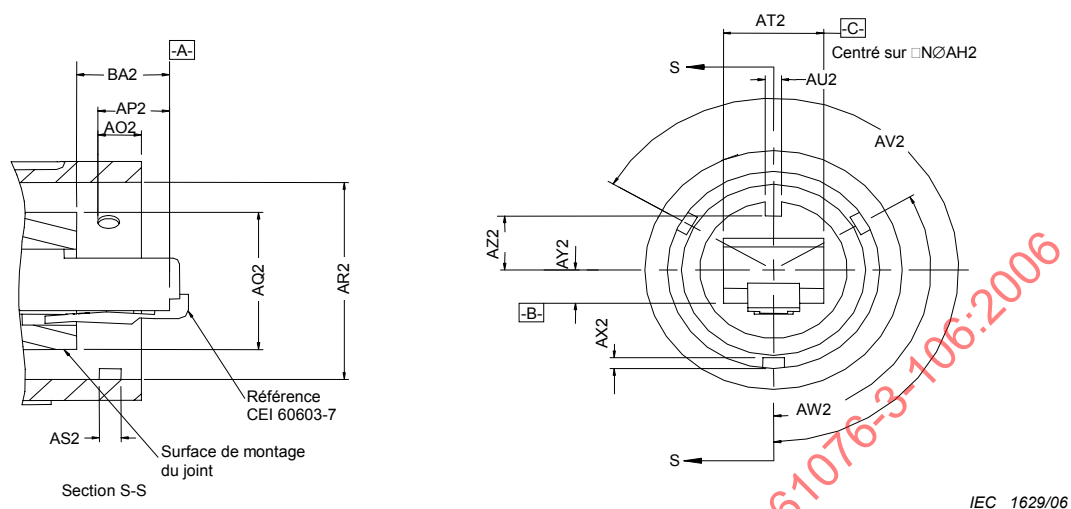
Figure 2 – Fiche, Variante 01
