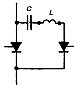
Figure A.1b – Circuit de commutation Exemple
