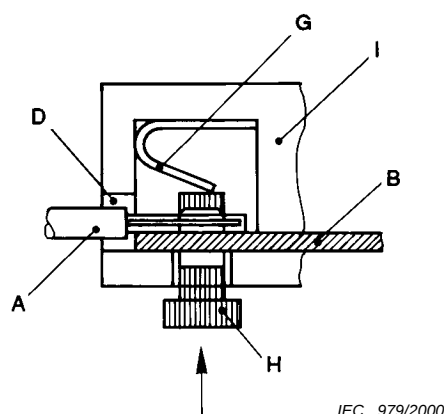
Figure 6a – Bornes sans vis avec organe de serrage à pression indirecte et desserage par un poussoir
