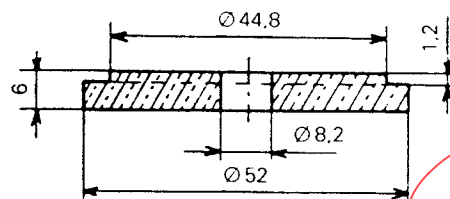
Laiton (B) Brass
