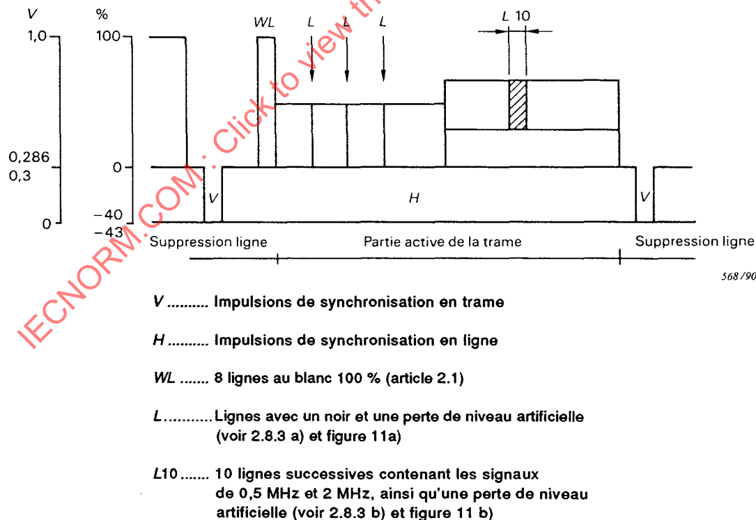
Figure 11c - Signal d'essai pour la mesure de la compensation des pertes de niveau luminance (préenregistré sur une bande d'essai)
