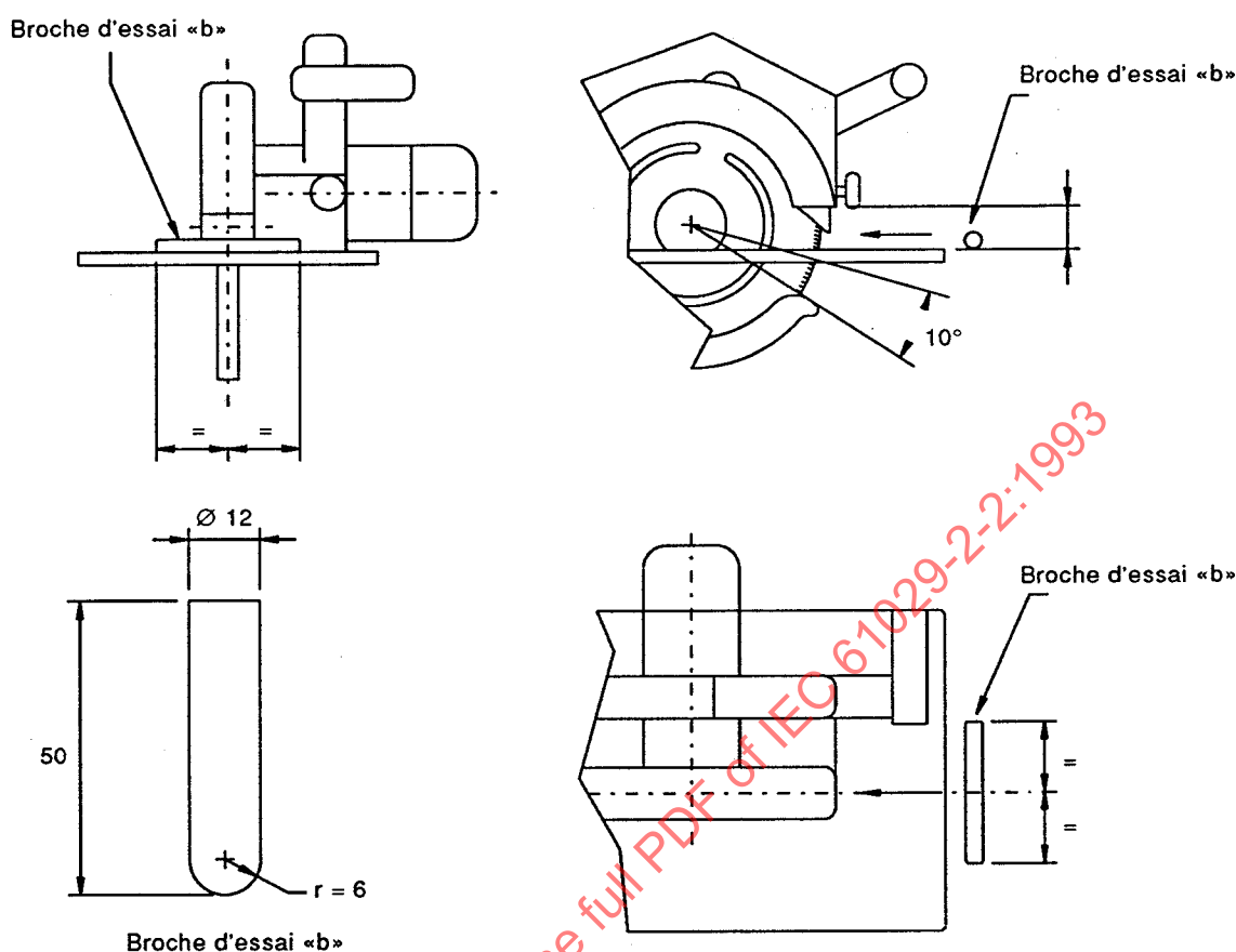
Figure 102 – Broche d'essai «b»
