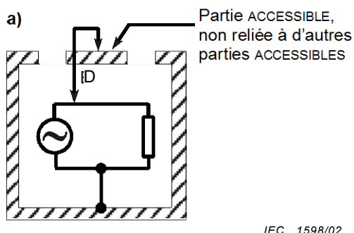
Figure D.2a) et Figure D.2b) – Protection entre un circuit interne sous TENSION DANGEREUSE et une partie ACCESSIBLE qui n'est pas reliée à d'autres parties ACCESSIBLES
