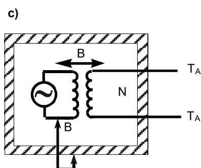
Figure D.2c) et Figure D.2d) – Protection entre des circuits primaires sous TENSION DANGEREUSE et des circuits qui ont des BORNES externes ACCESSIBLES
