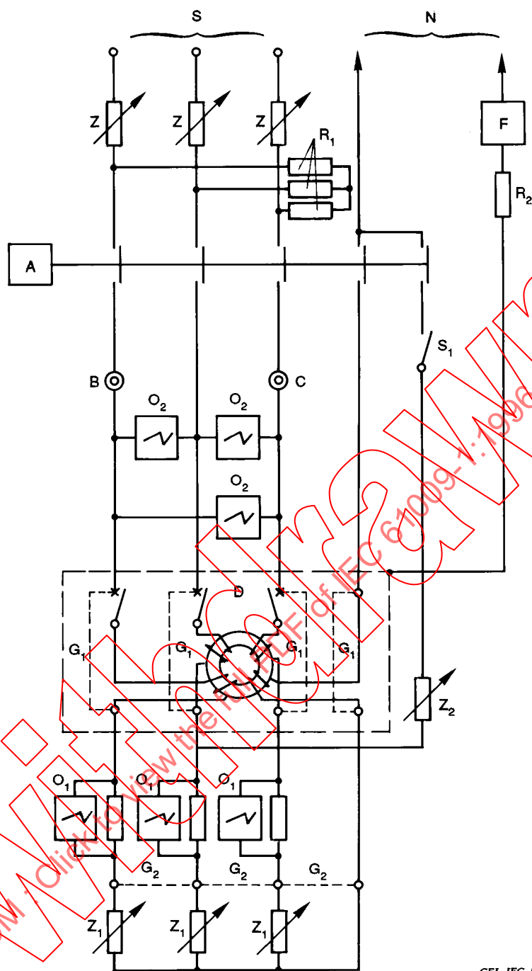
Figure 8 – Circuit d'essai pour la vérification du pouvoir de coupure assigné d'un DD tripolaire à quatre voies de courant, dans le cas d'un circuit triphasé avec neutre (9.12)
