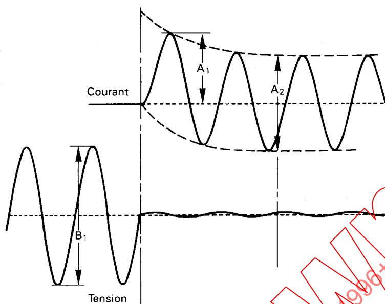
Figure 10 – Exemple d'enregistrement d'étalonnage pour essai de court-circuit
