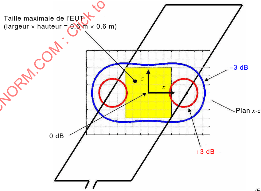
Figure B.6 – Isolignes +3 dB et -3 dB pour l'intensité du champ magnétique (amplitude) dans le plan x-z pour la bobine d'induction de 1 m × 2,6 m sans plan de masse de référence
