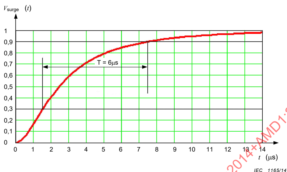
Figure E.8 – Tension de choc (10/700 μs): réponse de temps de montée T
