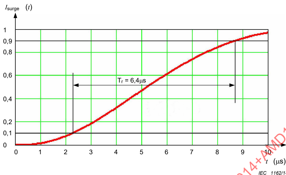
Figure E.5 – Courant de choc (8/20 \mu\text{s} ): réponse de temps de montée T_r
